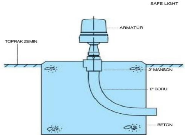
2" DEVE BOYNU MONTAJI
